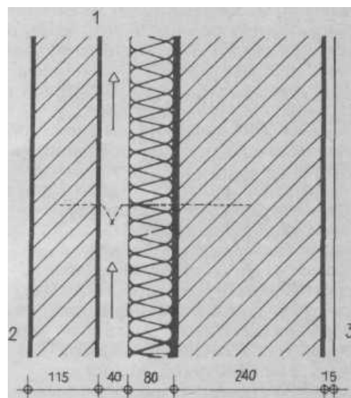
Рис. 7.13. Двухслойная наружная стена из кирпича с теплоизоляцией. Толщина воздушной прослойки 40 мм. Облицовочная стенка прикреплена к основной кладке анкерами 1 - наружная часть стены с вентилярованием; 2 — наружная сторона; 3-внутренняя сторона
