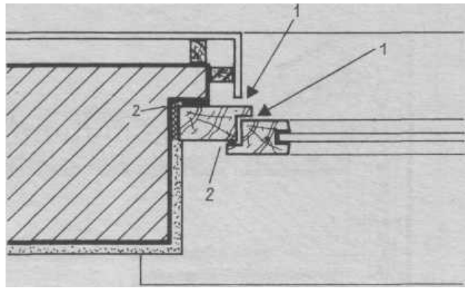
Рис. 7.15. Двухступенчатое уплотнение. Наружная облицовка стены образует внешнюю ступень стыка стены с окном, а шлиц глубиной 2-3 мм на раме - внешнюю ступень уплотнения рамы со створкой. Дождевая вода не проникает через эти уплотнения 1 - открытый стык; 2 - уплотнитель
